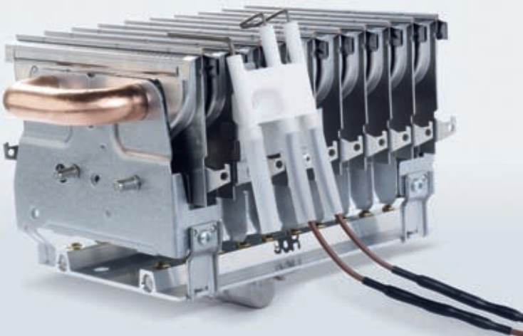
Quemador refrigerado
